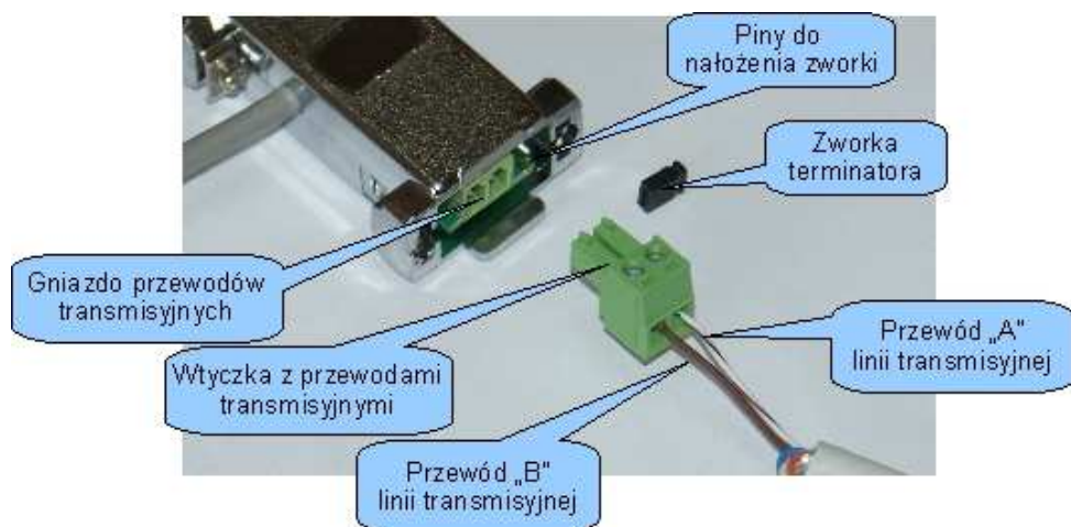
Rysunek 3 Podłączenie linii transmisyjnej do portu RS485 konwertera
