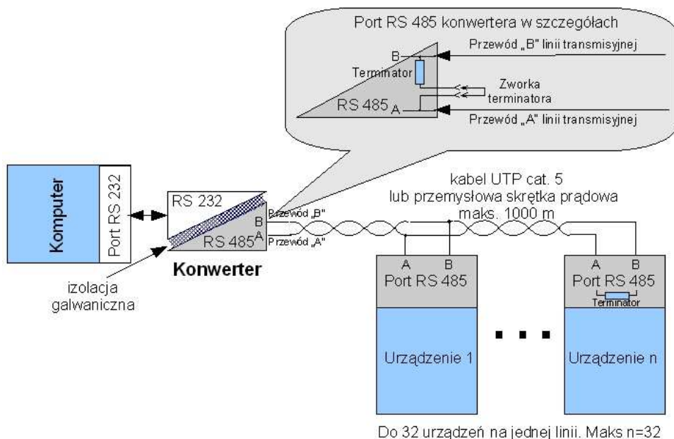
Rysunek 1 Schemat systemu transmisyjnego RS 232 / RS 485
